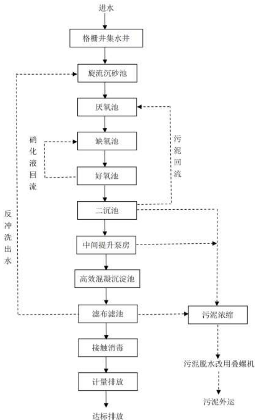
图 2-1 东海县驼峰乡联村生活污水处理厂污水处理工艺流程
