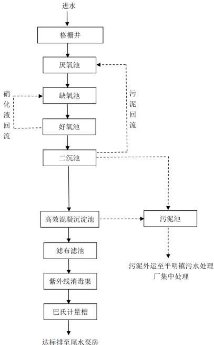
图 2-1 东海县张湾乡后湾村生活污水处理厂污水处理工艺流程
