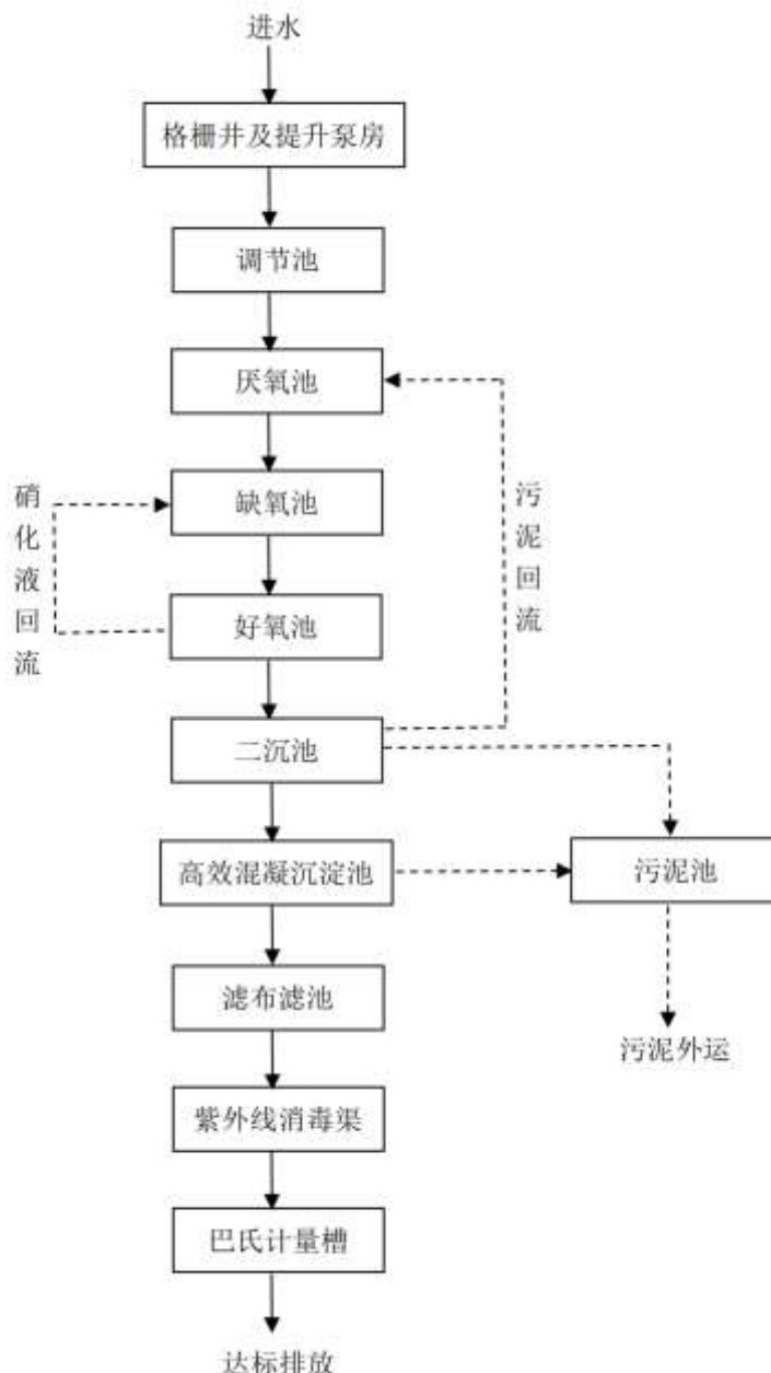
图 2-1 东海县石湖乡污水处理厂污水处理工艺流程
