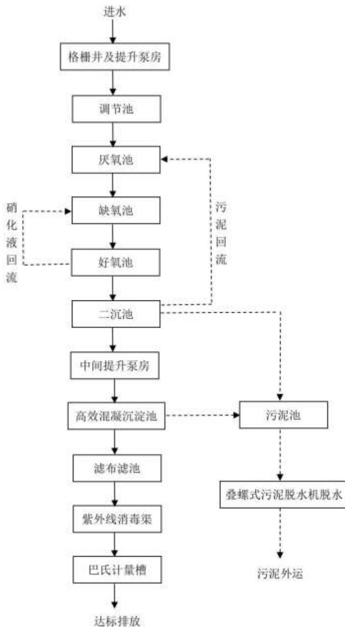
图 2-1 东海县平明镇污水处理厂污水处理工艺流程
