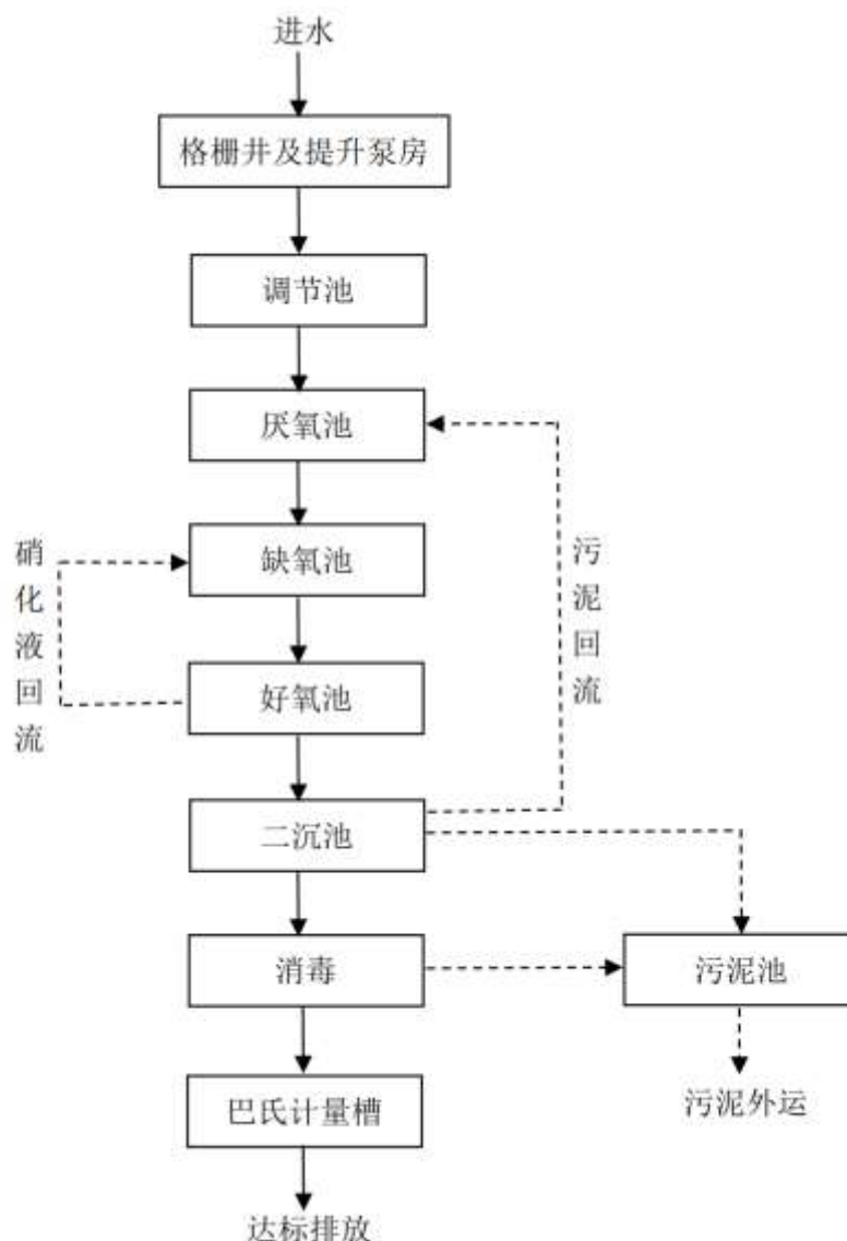
图 2-1 东海县青湖镇联村污水处理厂污水处理生产工艺流程 工艺流程简述
